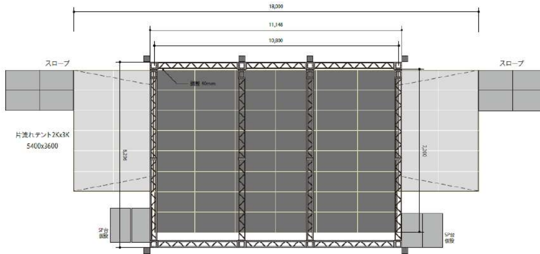
■平面図
