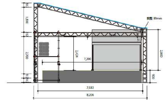
■側面図
