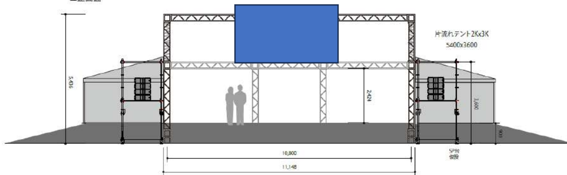
■正面図
